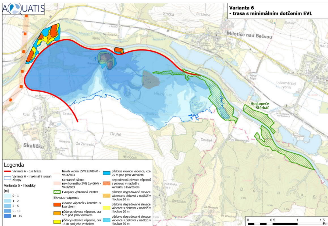
Obr. 8 Situace varianty V3.6 [14]
