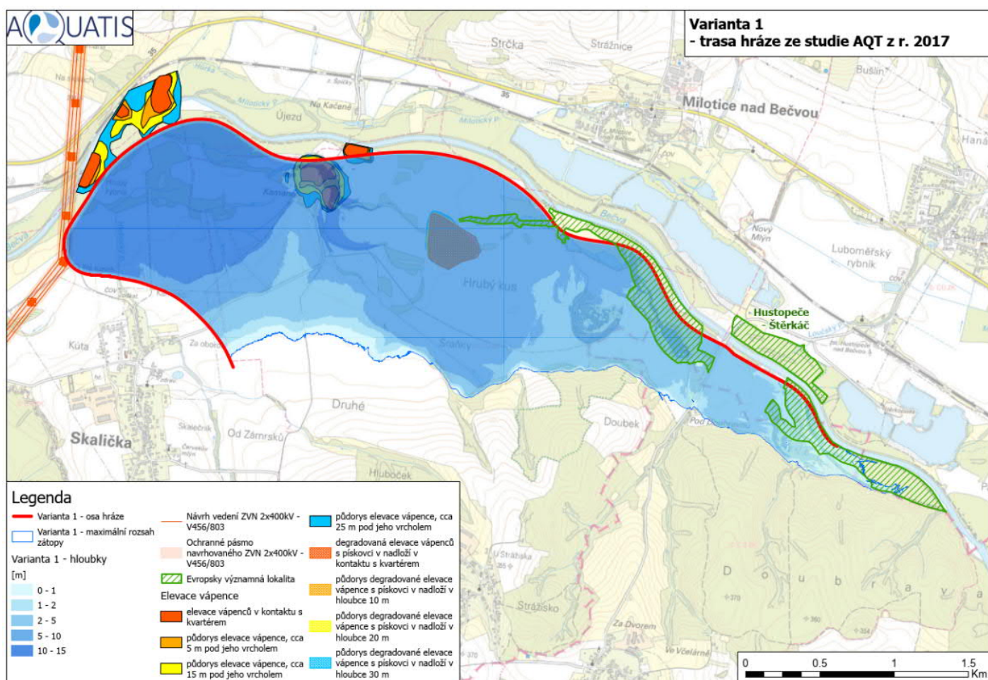
Obr. 3 Situace varianty V3.1 [14]
