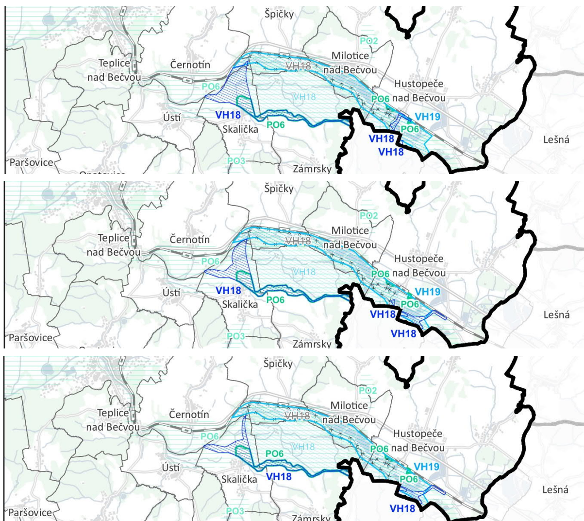
Obr. 1 Navrhované varianty boční suché nádrže Skalička v měřítku zpracování Z6b ZÚR OK (1:100 000). Shora dolů: VH18A, VH18B a VH18C
