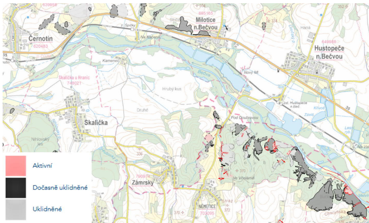
Obr. 31 Mapované svahové deformace v řešeném území a jeho okolí (ČGS, 2026)
