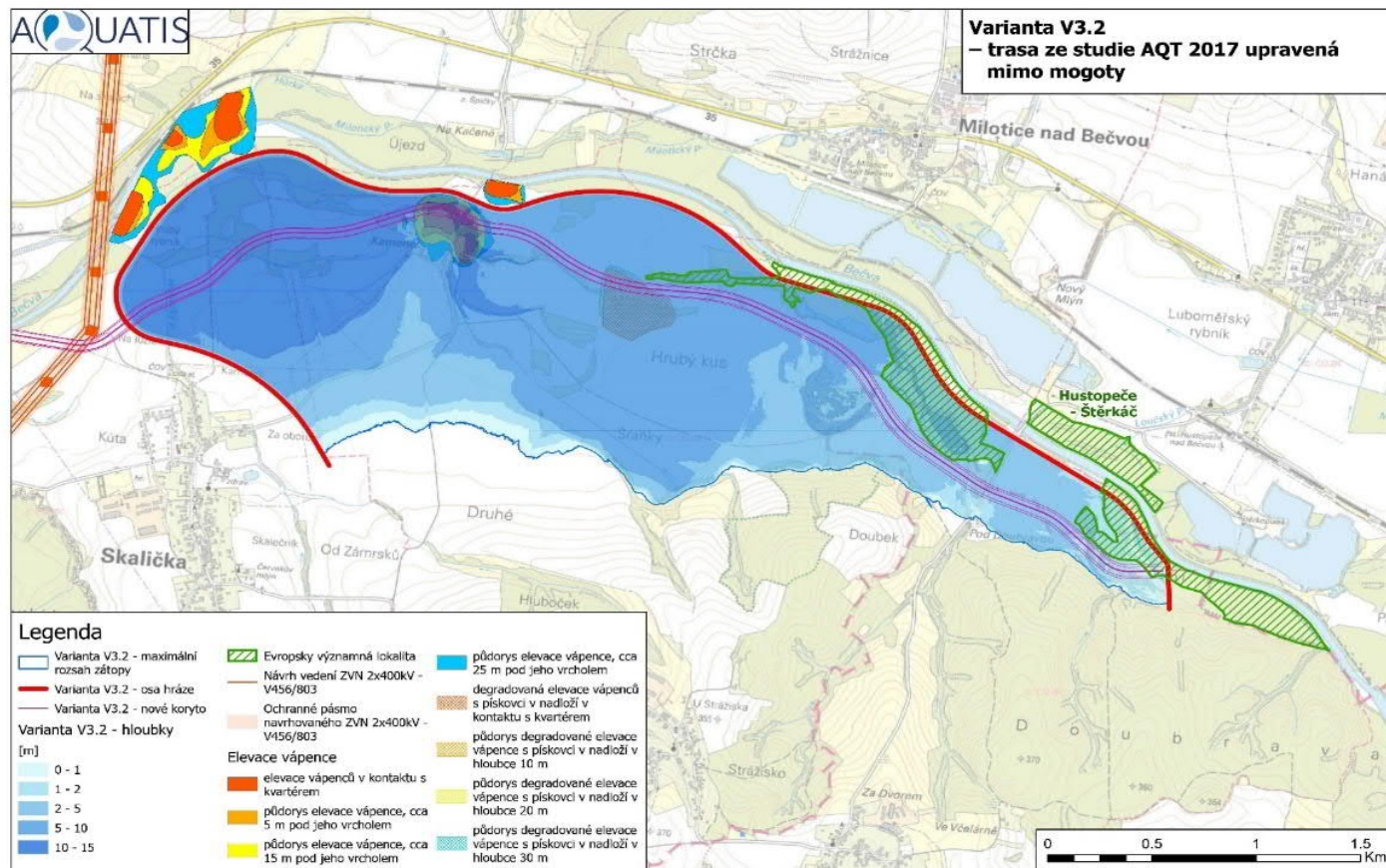
Obr. 4 Situace varianty V3.2 [14]
