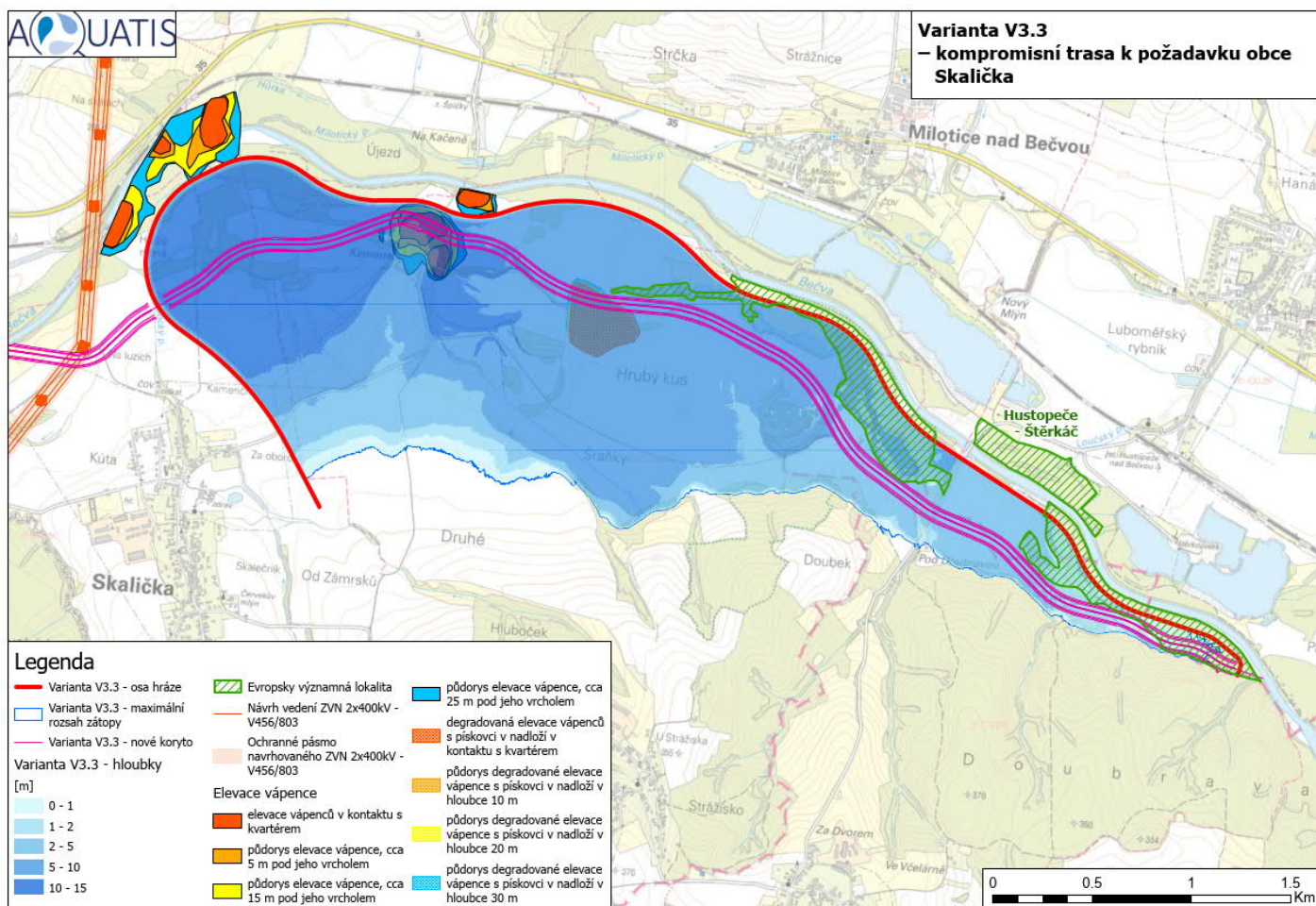
Obr. 5 Situace varianty V3.3 [14]
