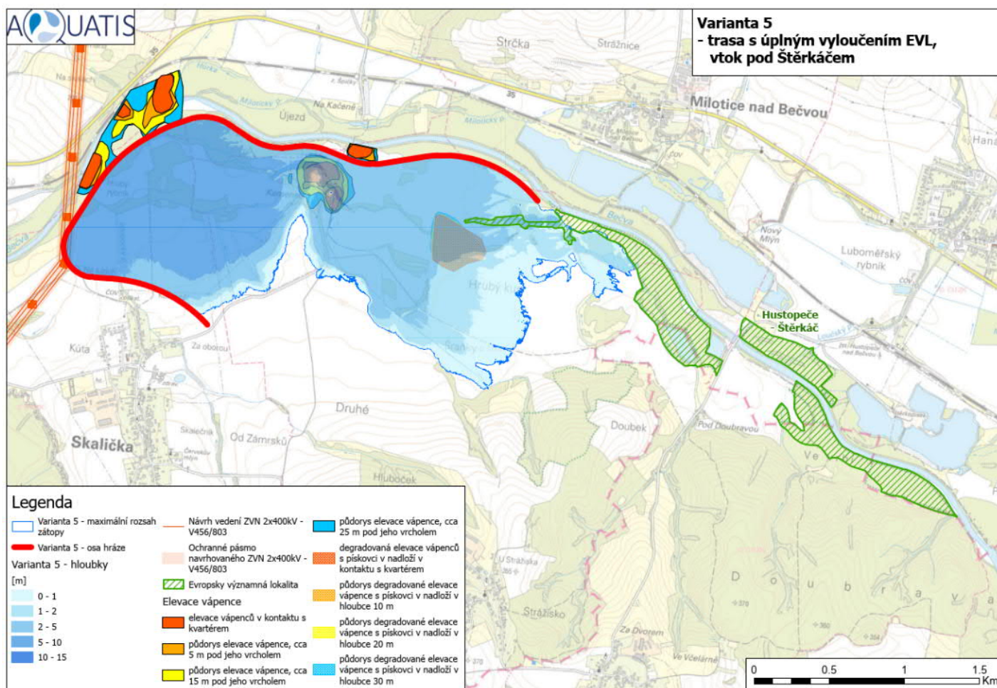
Obr. 7 Situace varianty V3.5 [14]
