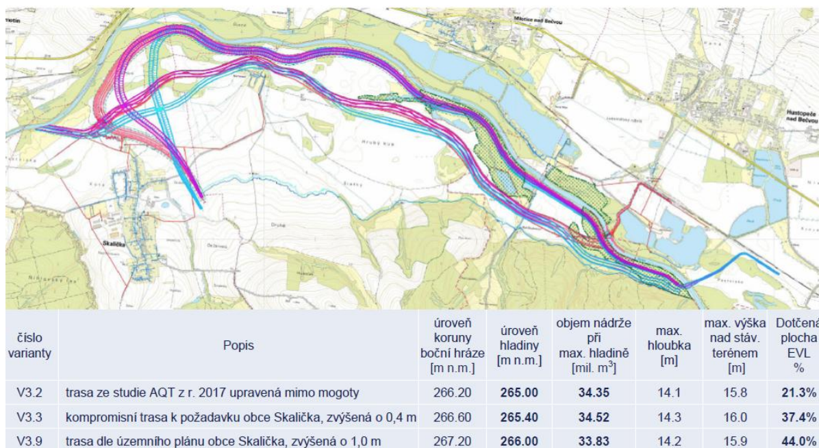
Obr. 1: Přehledná situace vymezení variant (Bečva, VD Skalička, předprojektová příprava, technické řešení, prezentace (Aquatris, 2025))
