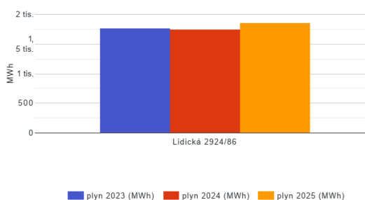
Spotřeba plynu areál Lidická 86, Prostějov (2023, 2024, 2025) (MWh)
