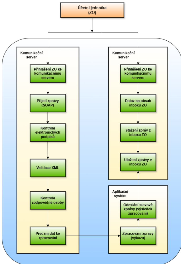
Obrázek 2: Schéma komunikace s CSÚIS
